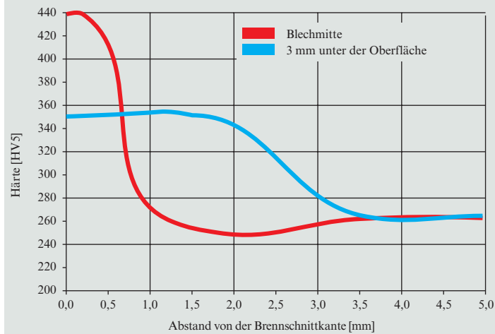
Bild 9: Typische Aufhärtung von DILLIMAX 690 an der Brennschnittkante beim Sauerstoff-Acetylen-Brennschneiden (Blechdicke: 20 bis 30 mm)
