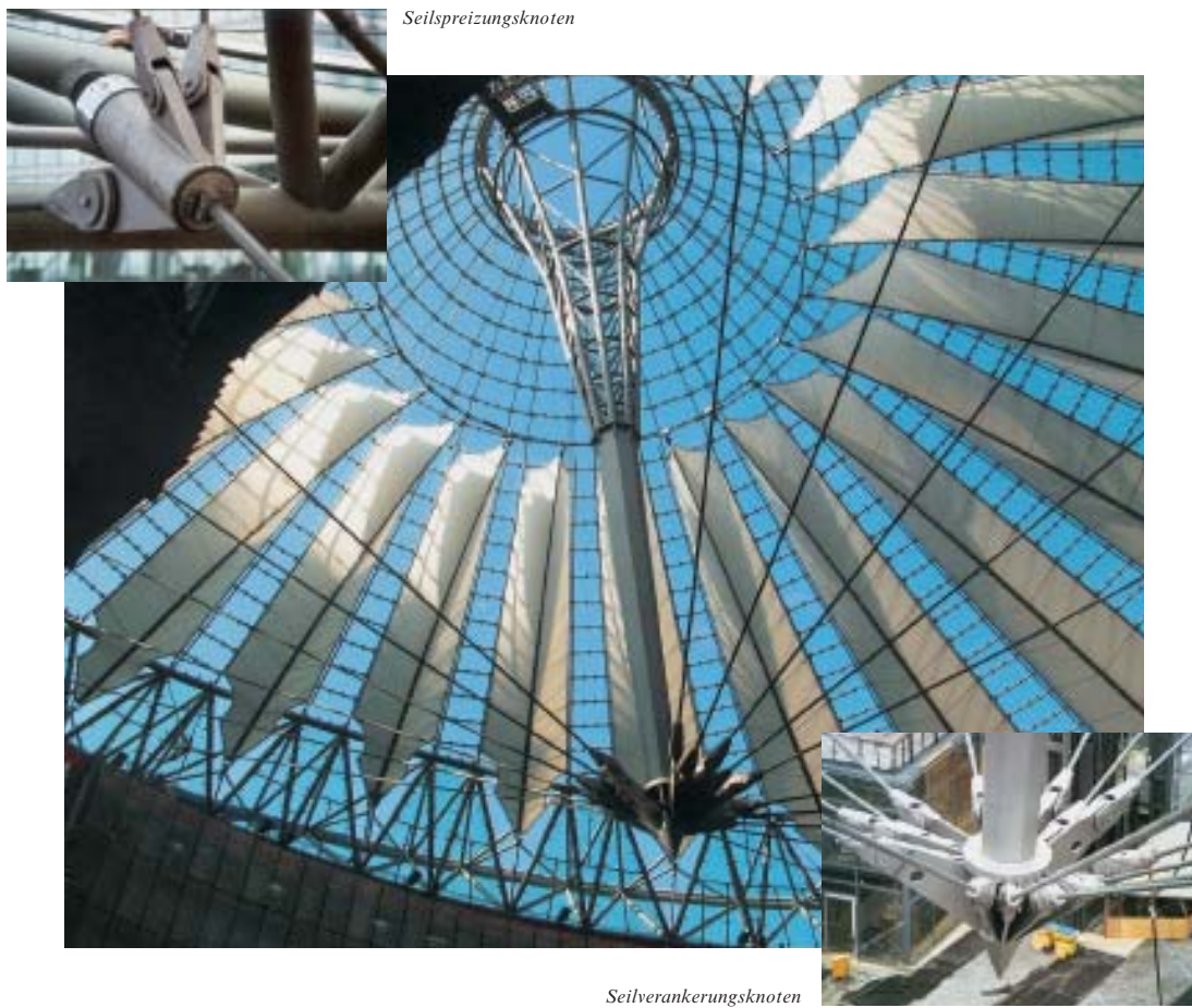
Bild 18: Dachkonstruktion des Sony-Center in Berlin, mit Laschen für den Ringbalken, die Seilspreizung- und Seilverankerungsknoten aus DILLIMAX 690 (Bild mit freundlicher Genehmigung von Waagner-Biró AG, Wien)
