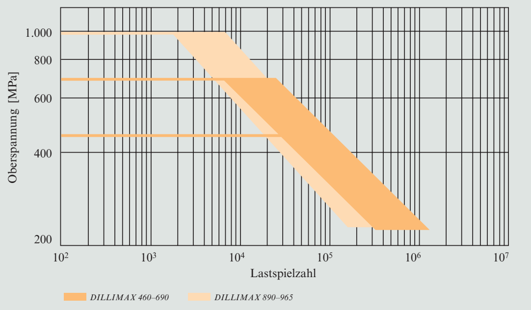
Bild 24: Wöhler-Streubänder von Schweißverbindungen aus DILLIMAX-Stählen (10 % bis 90 % Bruchwahrscheinlichkeit, V-Naht-Proben, 60°, Blechdicke 10 mm, R=0)
